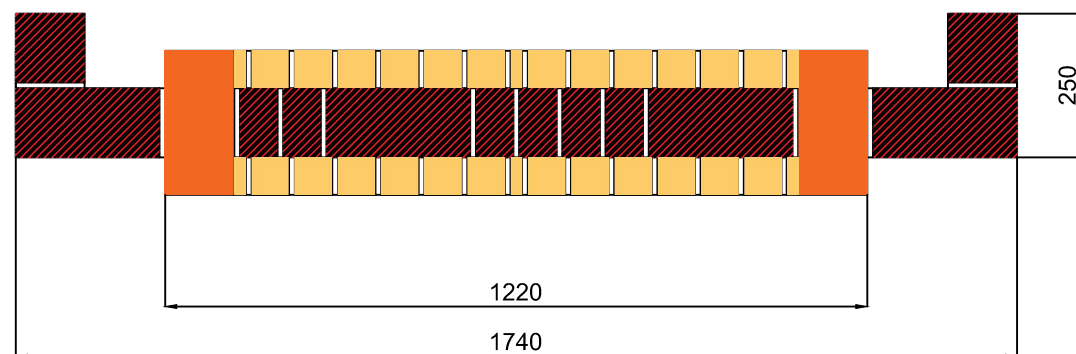
Огтлол 2-2
